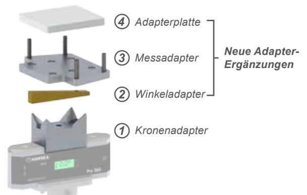
Neigungswinkelmesser mit 4 vers. Adaptern für unterschiedliche Mercedes-Benz Modelle.
