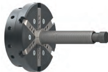
QuickHub geschlossen, max. Spannbereich 53,5 mm (ohne Erweiterungs-Aufsätze).
