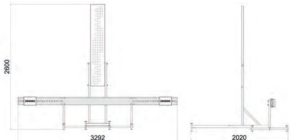
Schizzo con dimensioni (riflettore e traversa)
